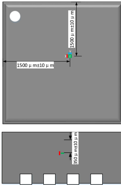
图 7-2. 各轴 Hall 元件在封装内的相对位置
