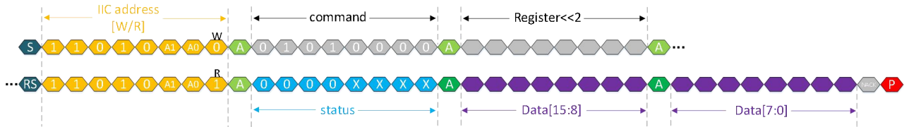
图 15-5. 读寄存器 I2C 时序图
