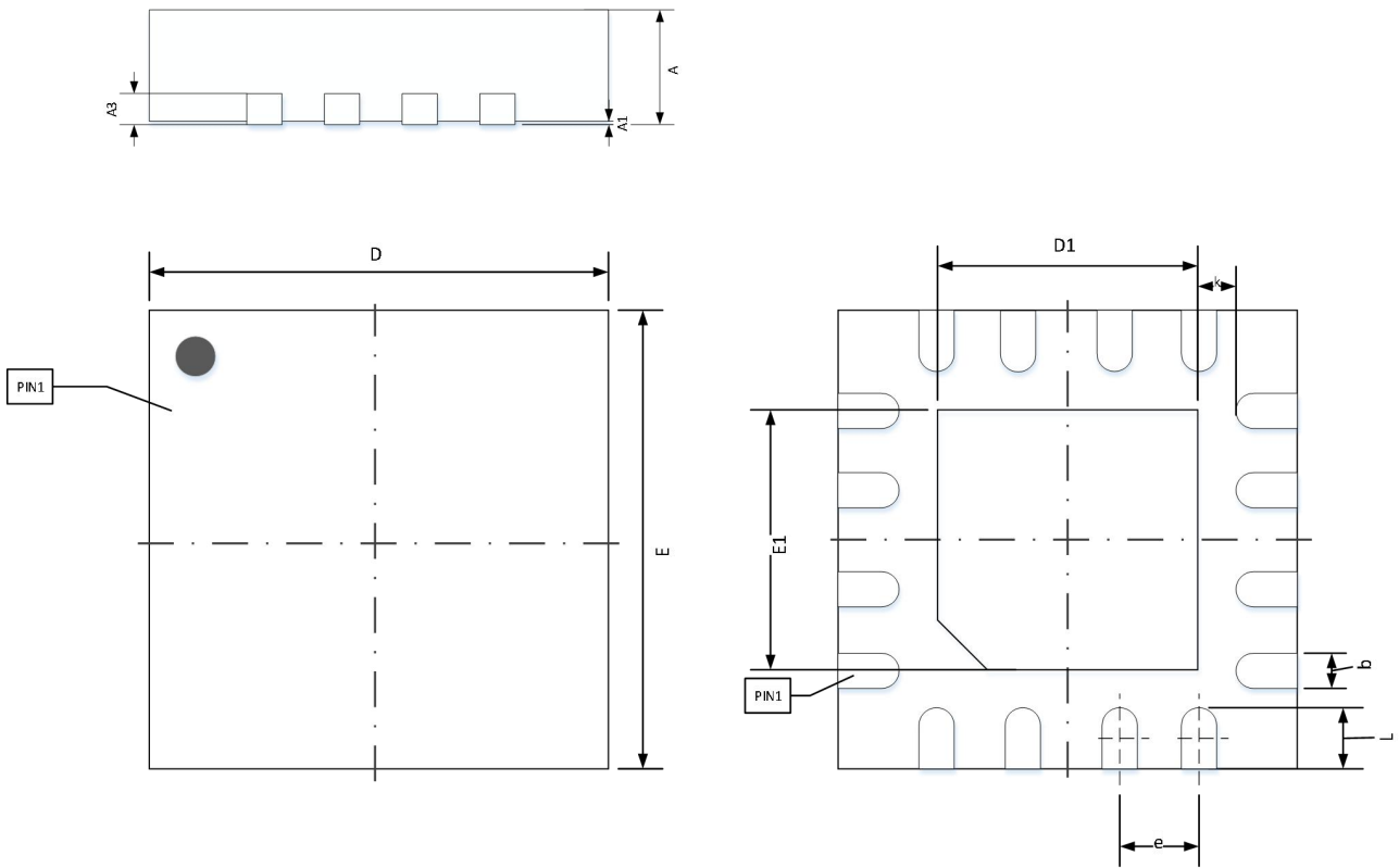
图 18-1. QFN_16PIN 封装尺寸图
