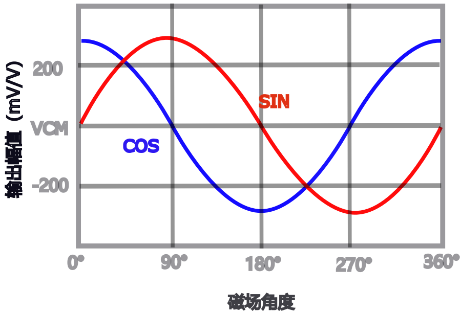
Figure 6: KTM5900 集成的 TMR 信号输出示意图
