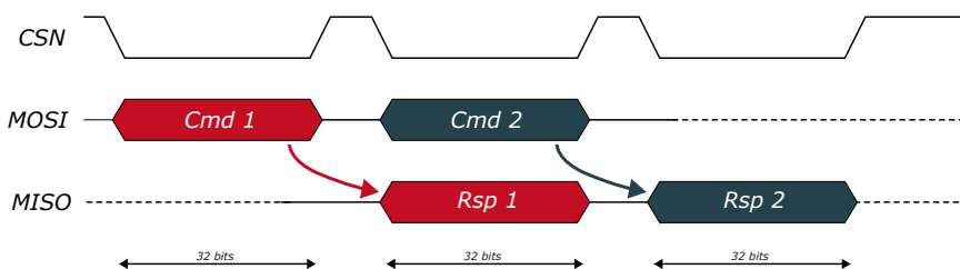
Figure 8: SPI 指令与回复时序示意图
